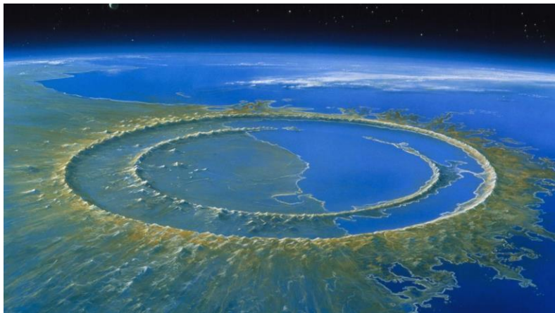
Кратер 150 км диаметра от столкновения с метеоритом 66 млн. лет до н.э. Юкатан, Мексика.
