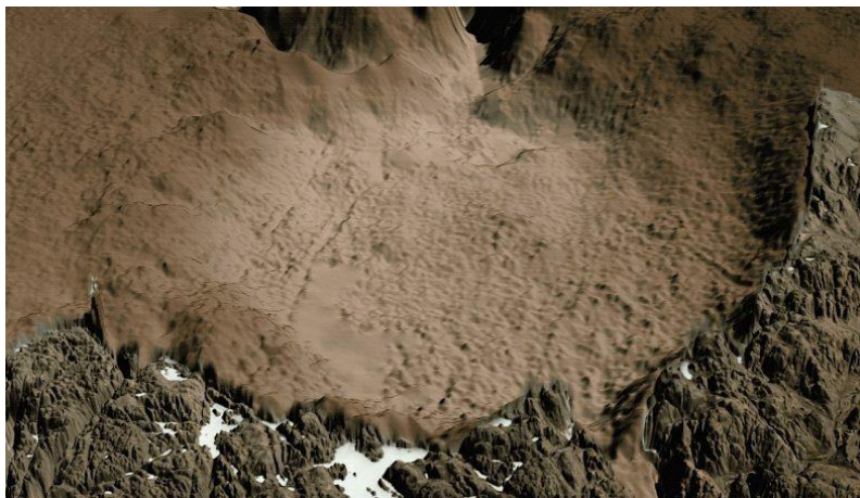
Кратер 30 км диаметра от столкновения с метеоритом, 12000 до н.э. Гренландия. Причина Younger Dryas оледенения? А может, причина потопа?
